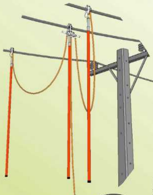
Grapa tipo "Pico Pato" Cat. FE-1192-CE
